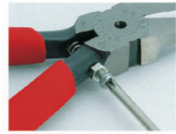
刃先が傷つかないように、調節可能なストッパー。
